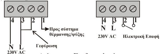
Διάγραμμα Συνδεσμολογίας
